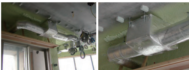
設置例
